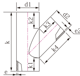
Y Branch 45°
