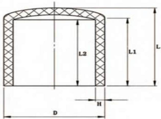
End Cap 2
